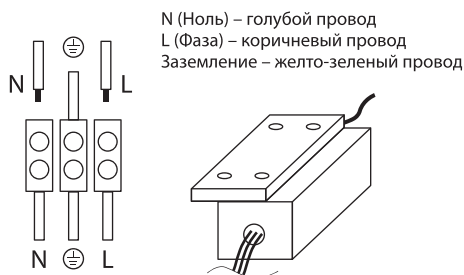
Рисунок 2. Этапы монтажа светильника SQ0358-0202
