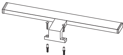
Рисунок 1. Этапы монтажа светильников SQ0358-0214, SQ0358-0215
